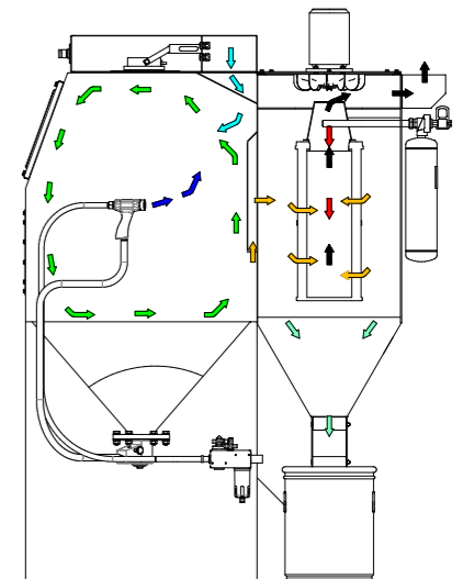
▼ Injectorstraalprincipe
